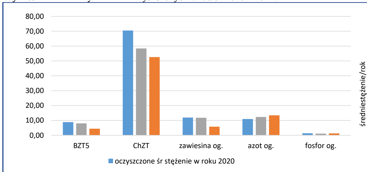
Wykres 24. Parametry ścieków oczyszczonych w latach 2020 – 2022.
