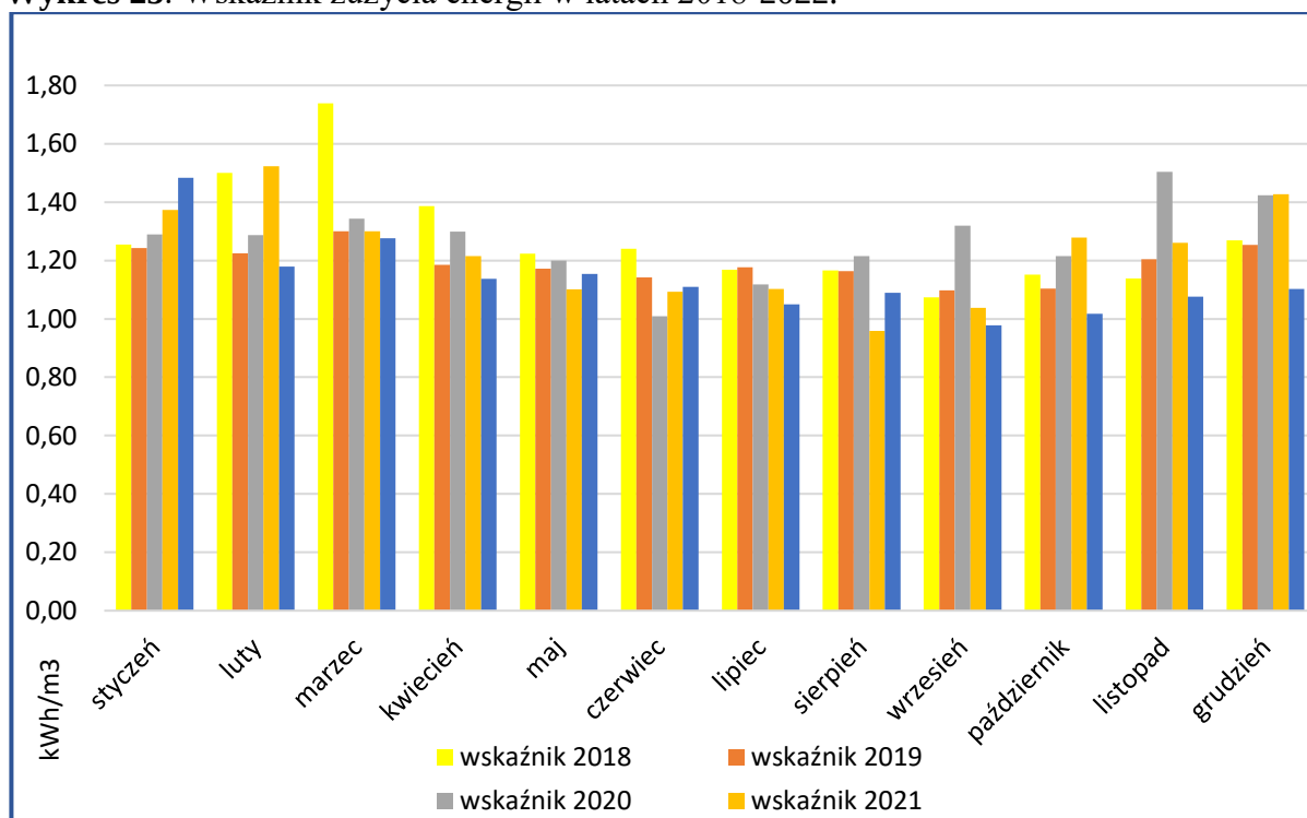
Wykres 25. Wskaźnik zużycia energii w latach 2018-2022.
