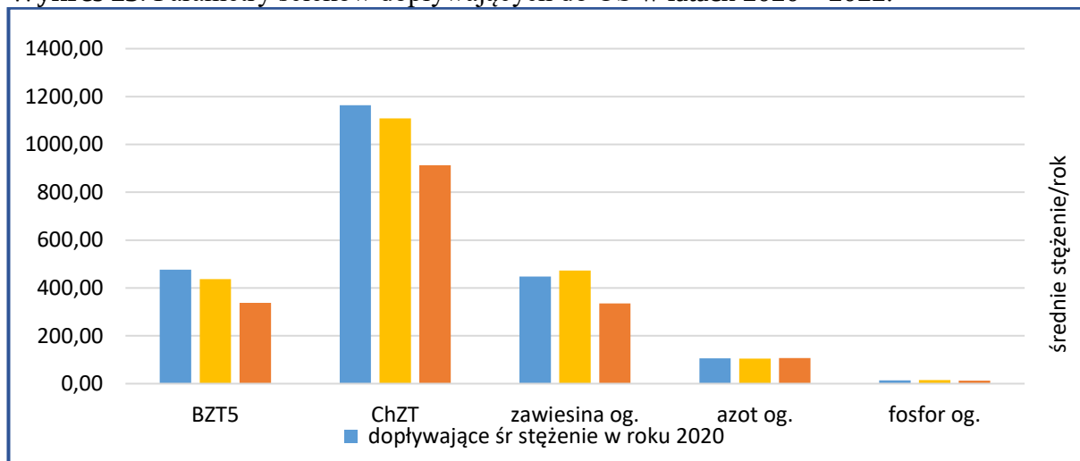
Wykres 23. Parametry ścieków dopływających do OŚ w latach 2020 – 2022.
